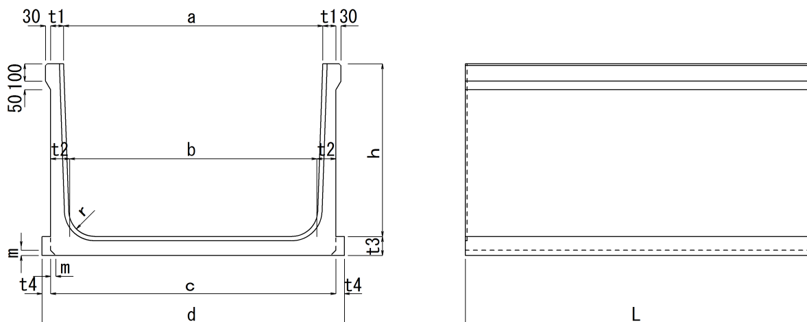
壁頂部水平線上の載荷重及び土質条件による区分
